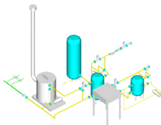
Fig 2: Vista 3-D del circuito di prova
